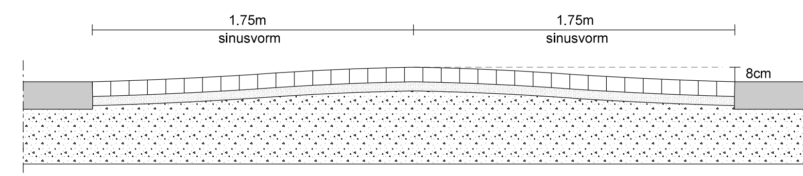
Drempelconstructie 1:20
