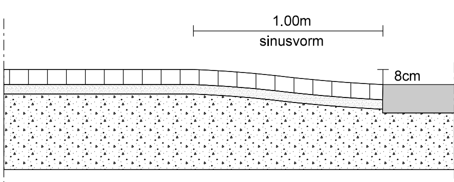
Plateauconstructie 1:20
